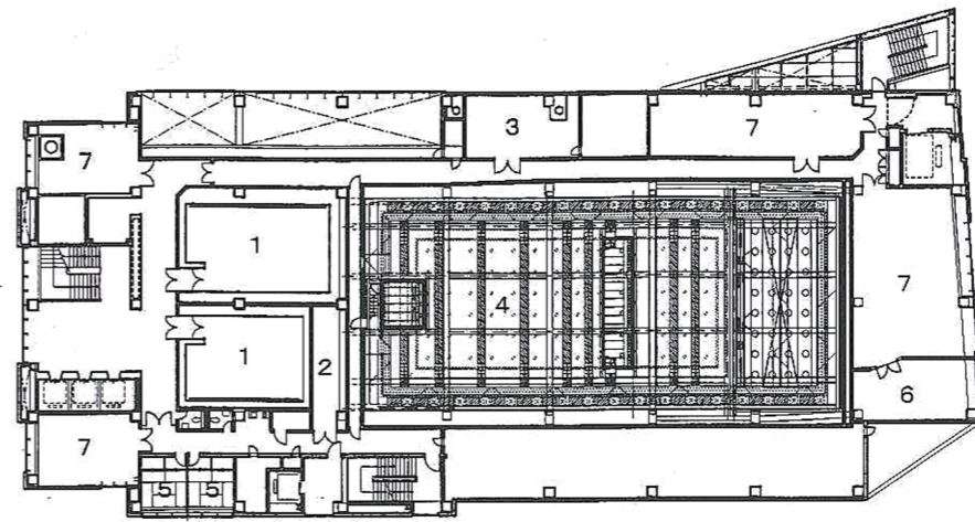
5階平面図
