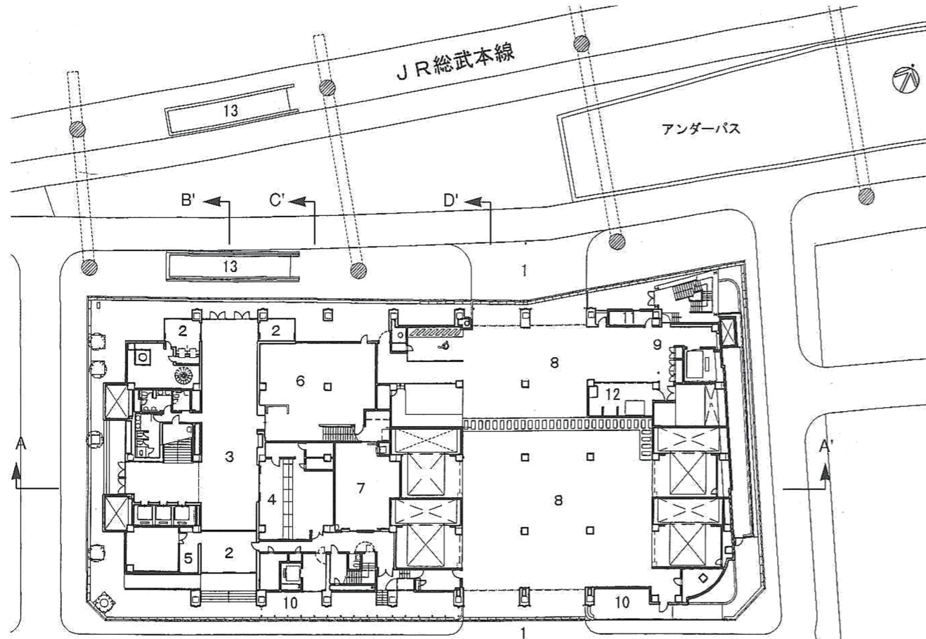
配置図・1階平面図
