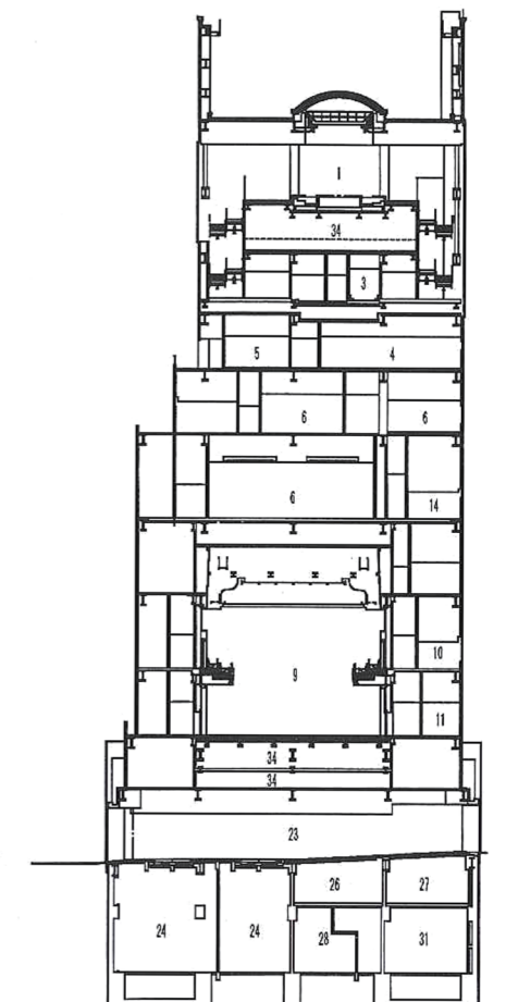
D-D'断面図
