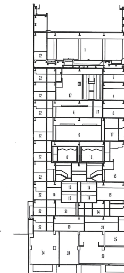
C-C'断面図
