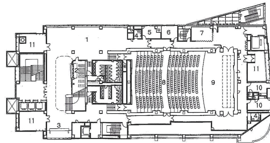
3階平面図
